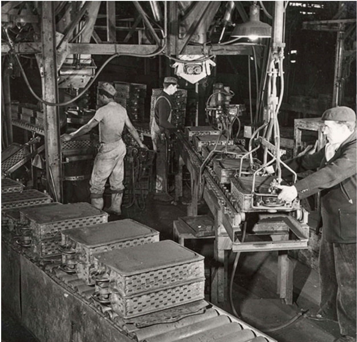
Fonderie. Machines à mouler Osborn.
