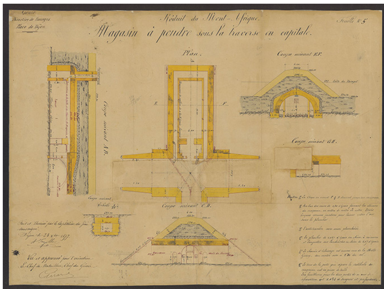
Réduit du Mont-Afrique. Magasin à poudre sous la traverse en capitale. 1877.
