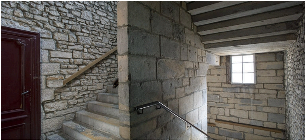
Détail de l'escalier principal en maçonnerie, avec la fenêtre éclairant la cage.
