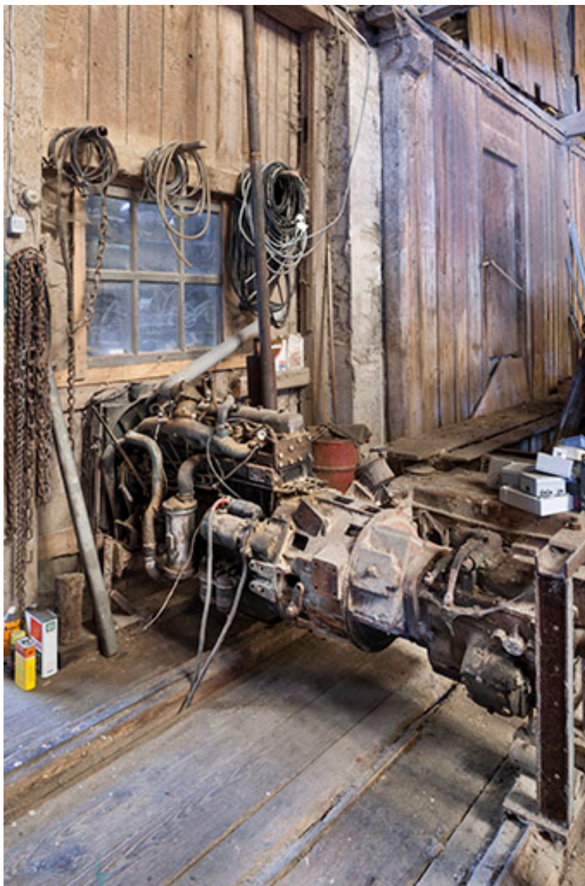
Moteur auxiliaire Saviem.
