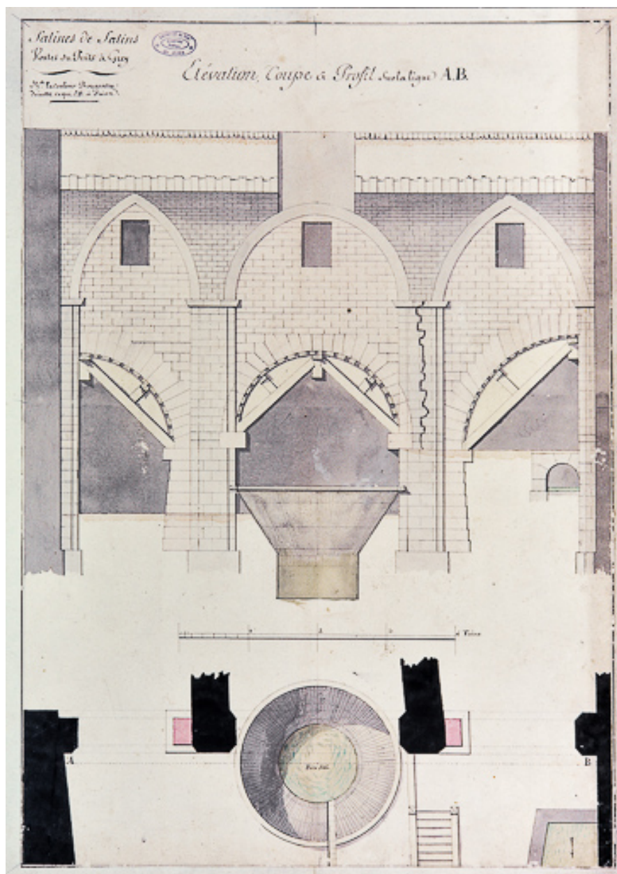
Voutes du Puits à Grey. Elévation. Coupe et profil sur la ligne A.B., s.d. [18e siècle].
