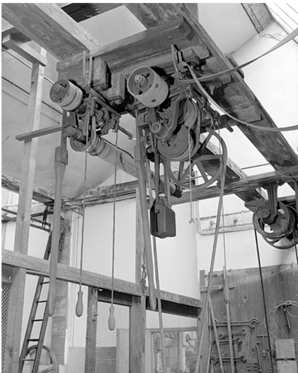
Détail du double système de transmission.
