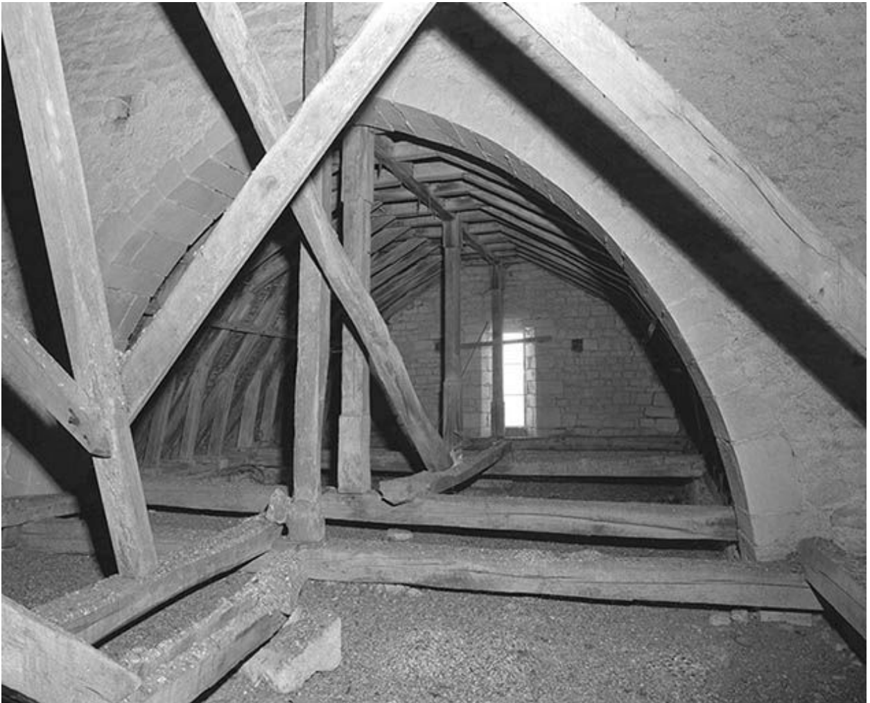
Comble : charpentes de la nef et du choeur.
