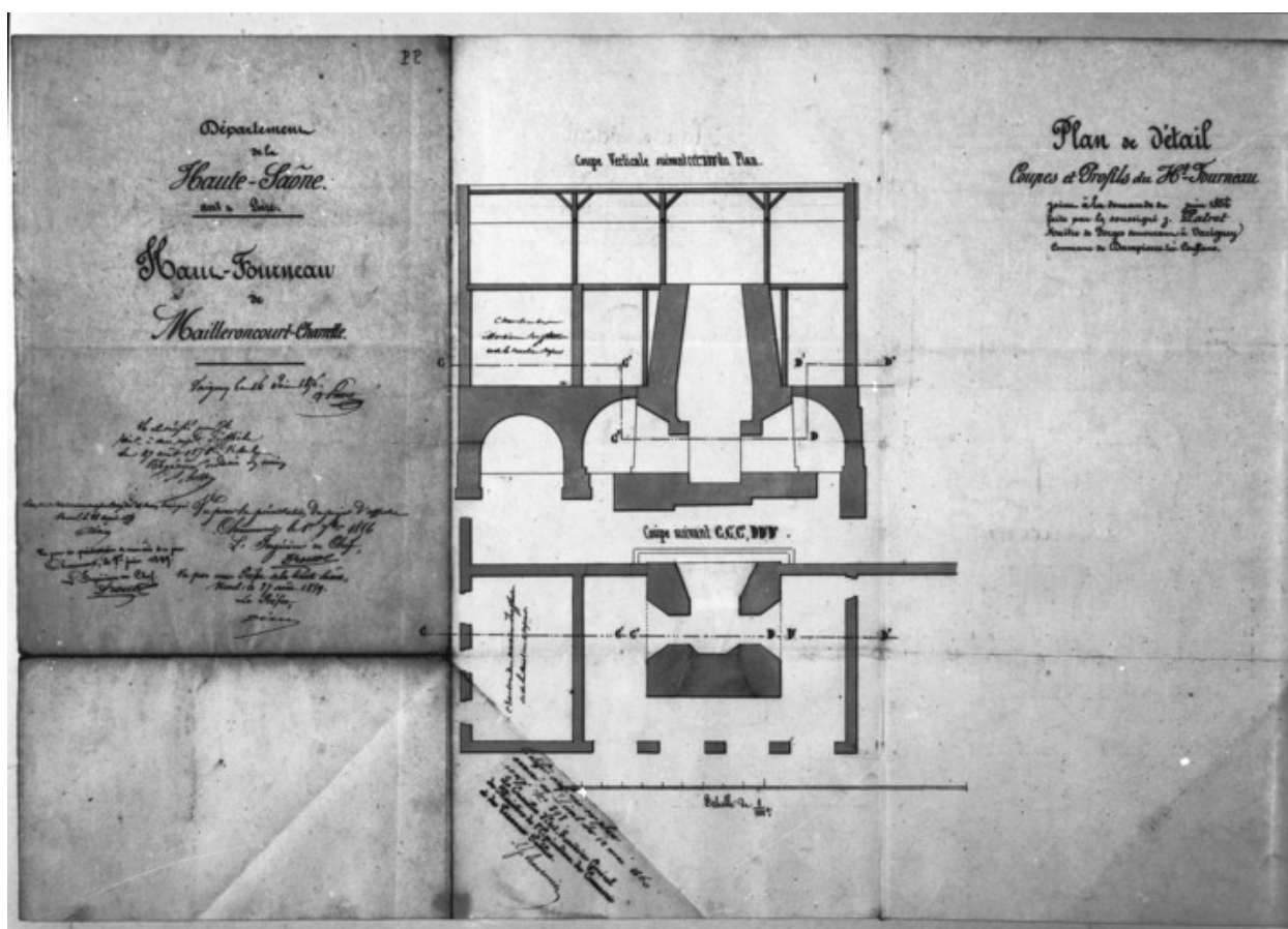
Haut fourneau de Mailleroncourt-Charrette. Plan de détail, coupes et profils du haut fourneau.
