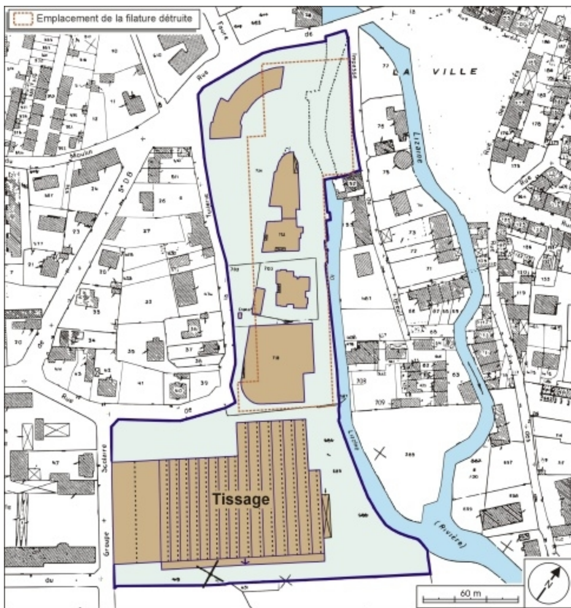
Plan-masse et de situation de l'usine. Extrait du plan cadastral numérisé, 2005, section AR, 1:1000 réduit à 1:2000.
