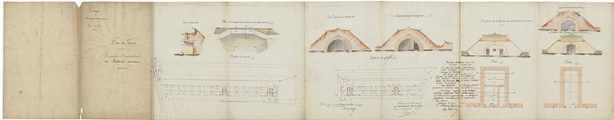
Fort de Varois. Croquis d'exécution des batteries annexes. 1880.
