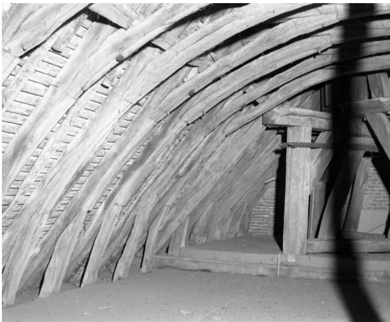
Charpente du comble
