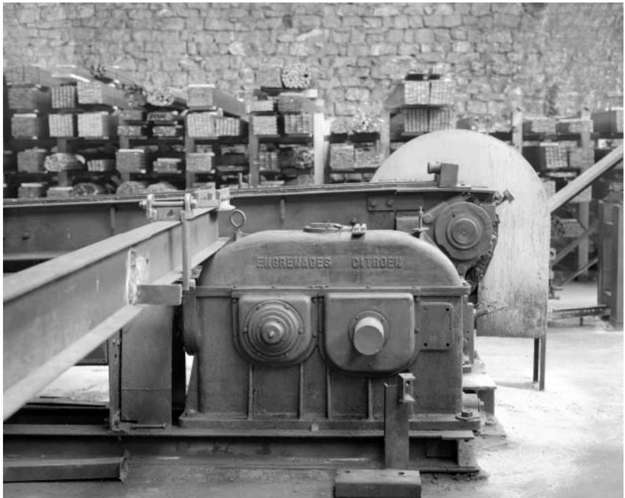
Banc d'étirage : système de transmission à engrenages Citroën.
