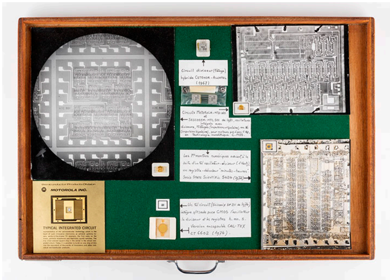
Circuits électroniques pour montre à quartz dont, en haut, un circuit diviseur hybride Cetehor-Alcatel (1967).
