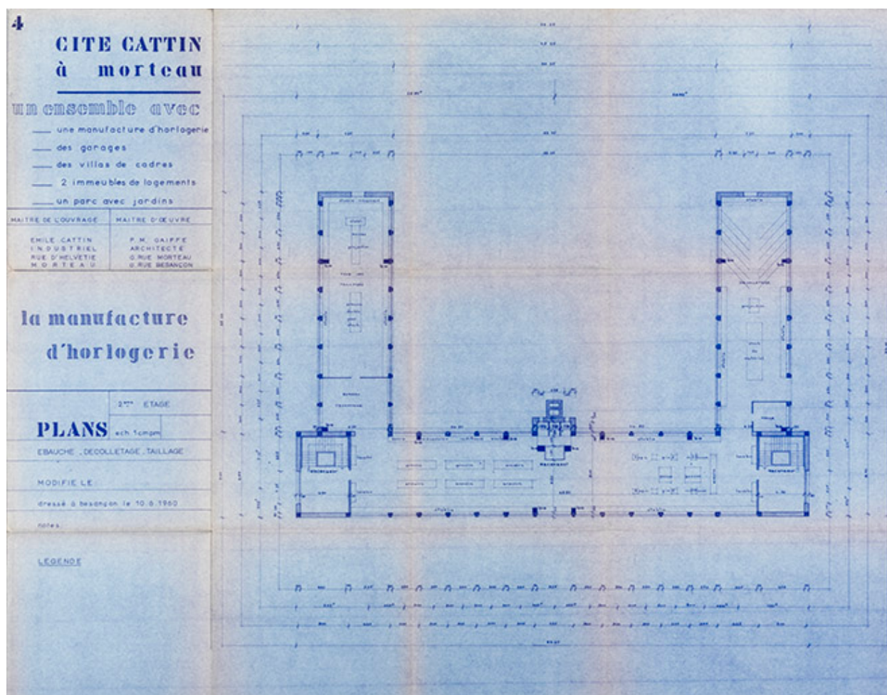
Cité Cattin à Morteau [...] 4. La manufacture d'horlogerie. Plans 2ème étage. Ebauche, décolletage, taillage, 10 juin 1960.
