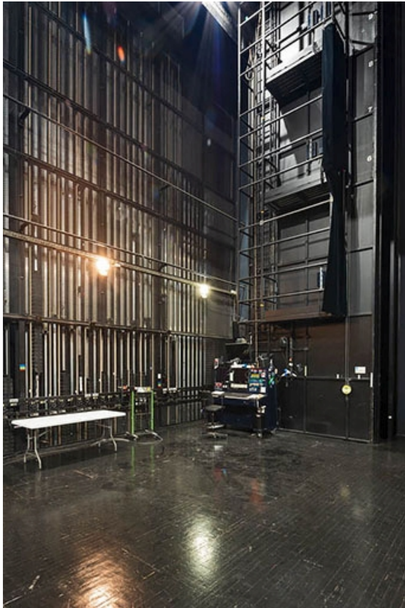
Cage de scène : fils de commande des perches en coulisse.
