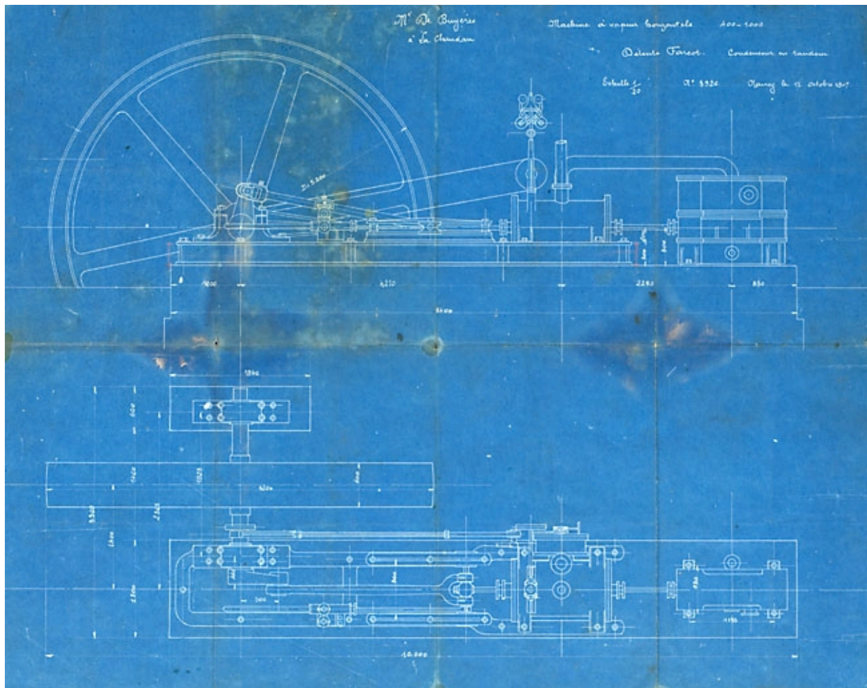
Machine à vapeur horizontale Farcot.
