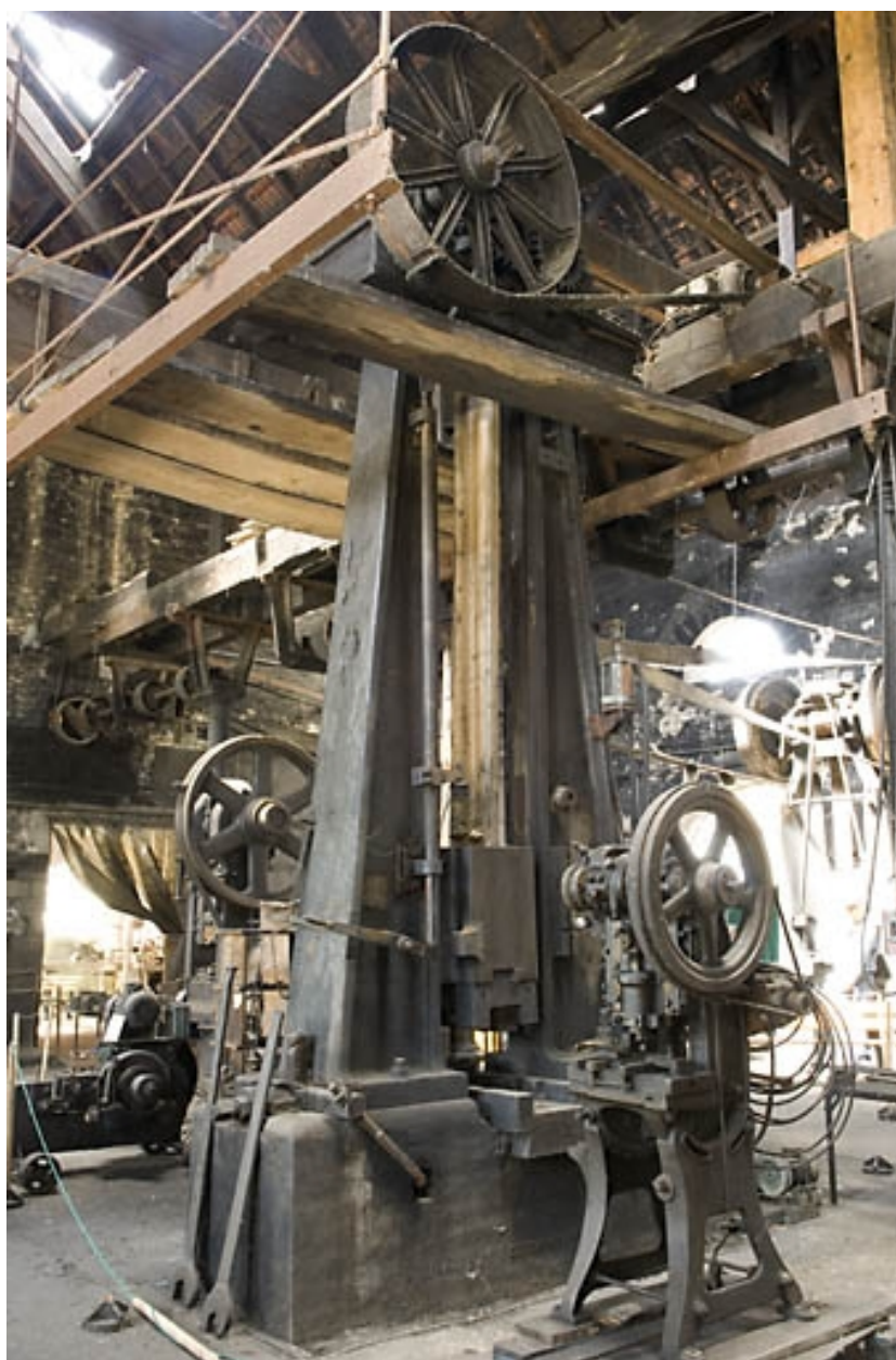
Atelier est. Marteau-pilon Olier et Cie (Clermont-Ferrand).
