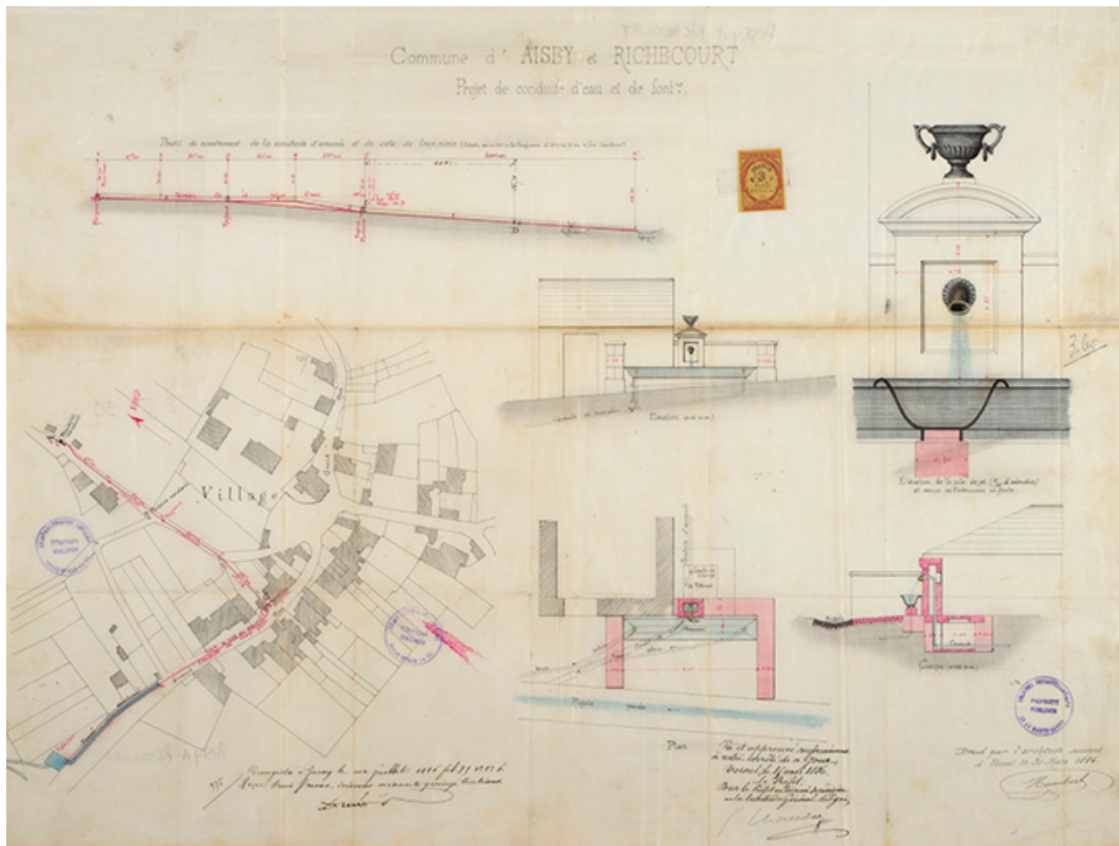
Projet de conduites d'eau et de fontaines, 1886.
