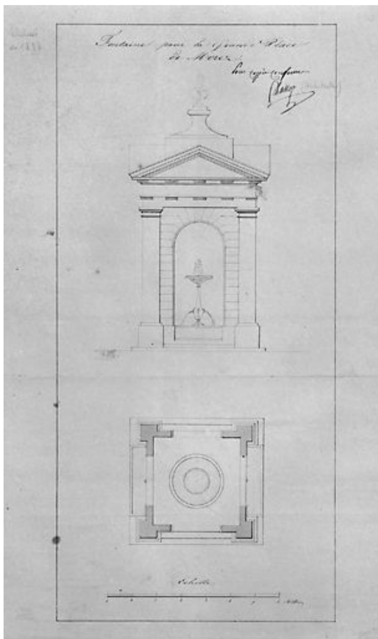
Fontaine pour la Grande Place de Morez [plan et élévation] : dessin (plume, lavis), s.d. [vers 1836], échelle approximative 1:70.
