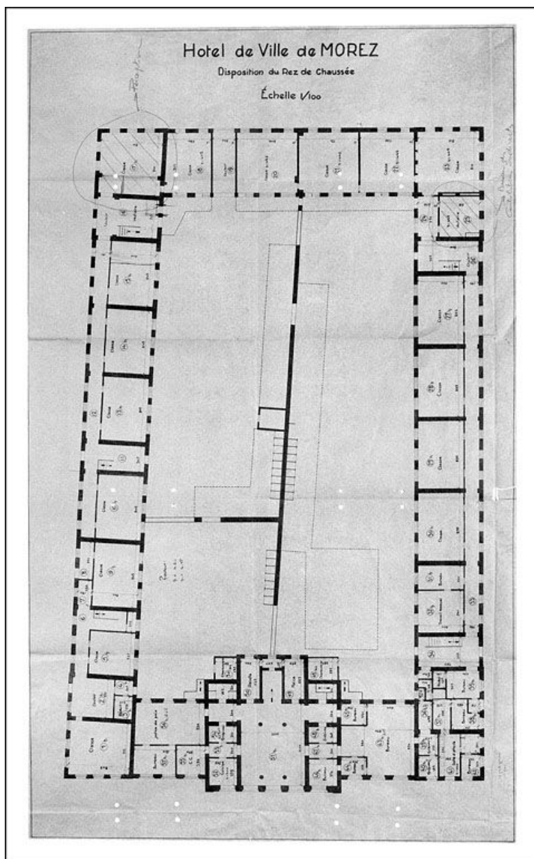
Hôtel de ville de Morez. Disposition du rez-de-chaussée, 2e quart 20e siècle.
