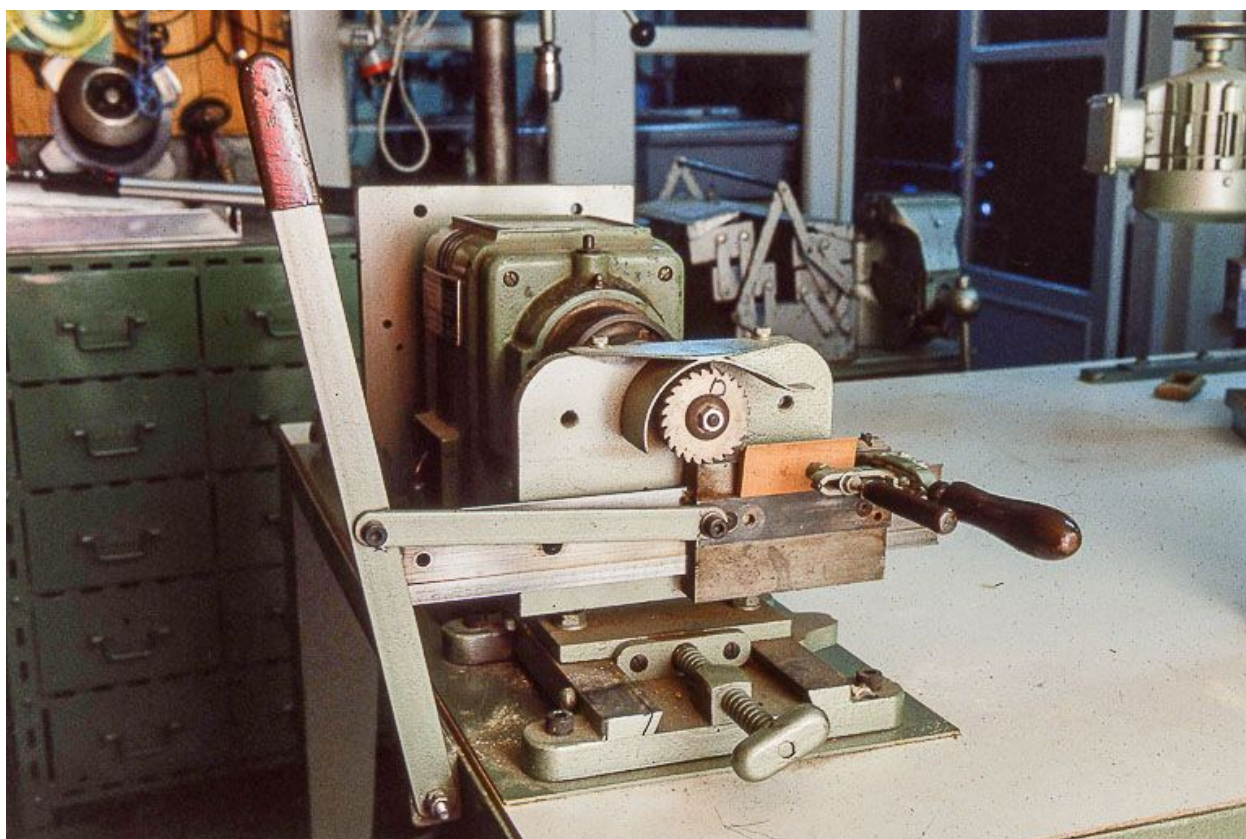
Détail de la fraise (côté fraiseuse).
