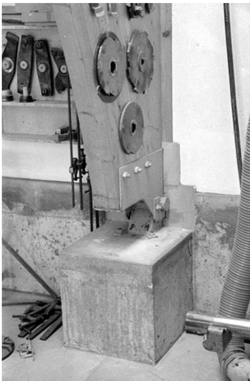
Support d'une ferme de la charpente.
