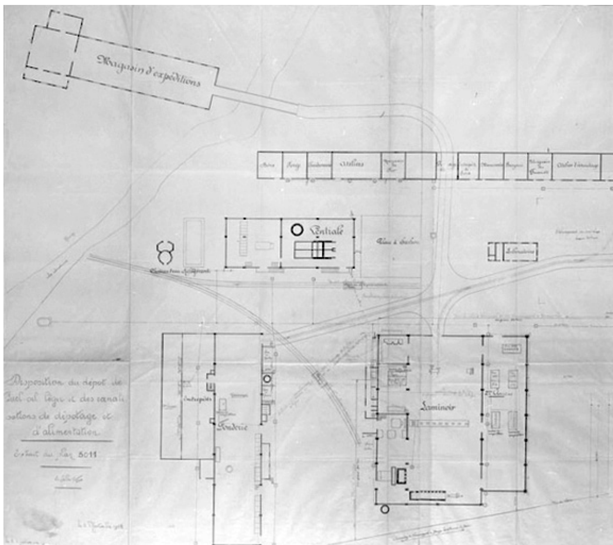
[Plan général des Aciéries].
