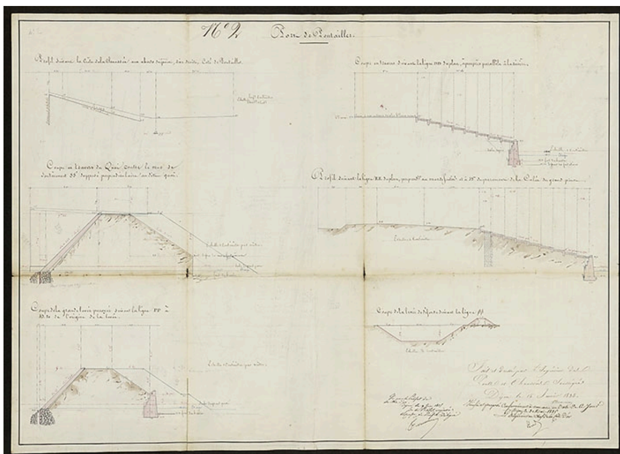
Port de Pontailier. [Coupes et profils]. 1835.
