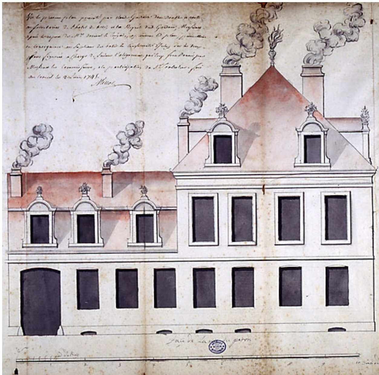
Elévation de la façade latérale gauche.
