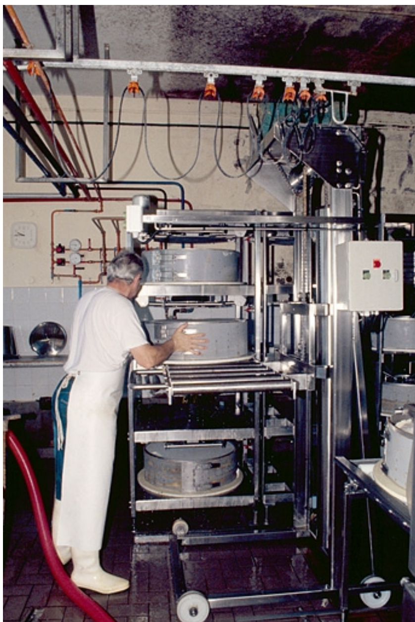
Mise en place d'un moule dans la presse hydraulique.
