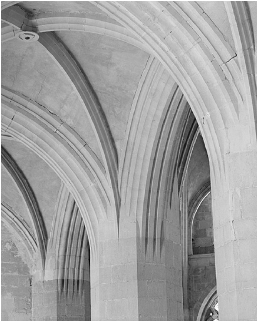
Retombées des nervures des voûtes des septième et huitième travées du collatéral nord.
