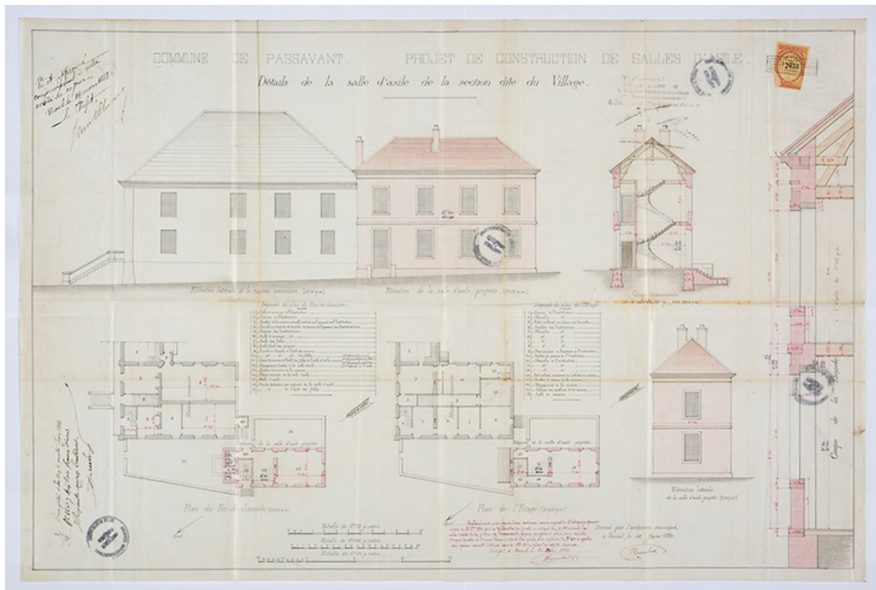
Projet de construction d'une salle d'asile.
