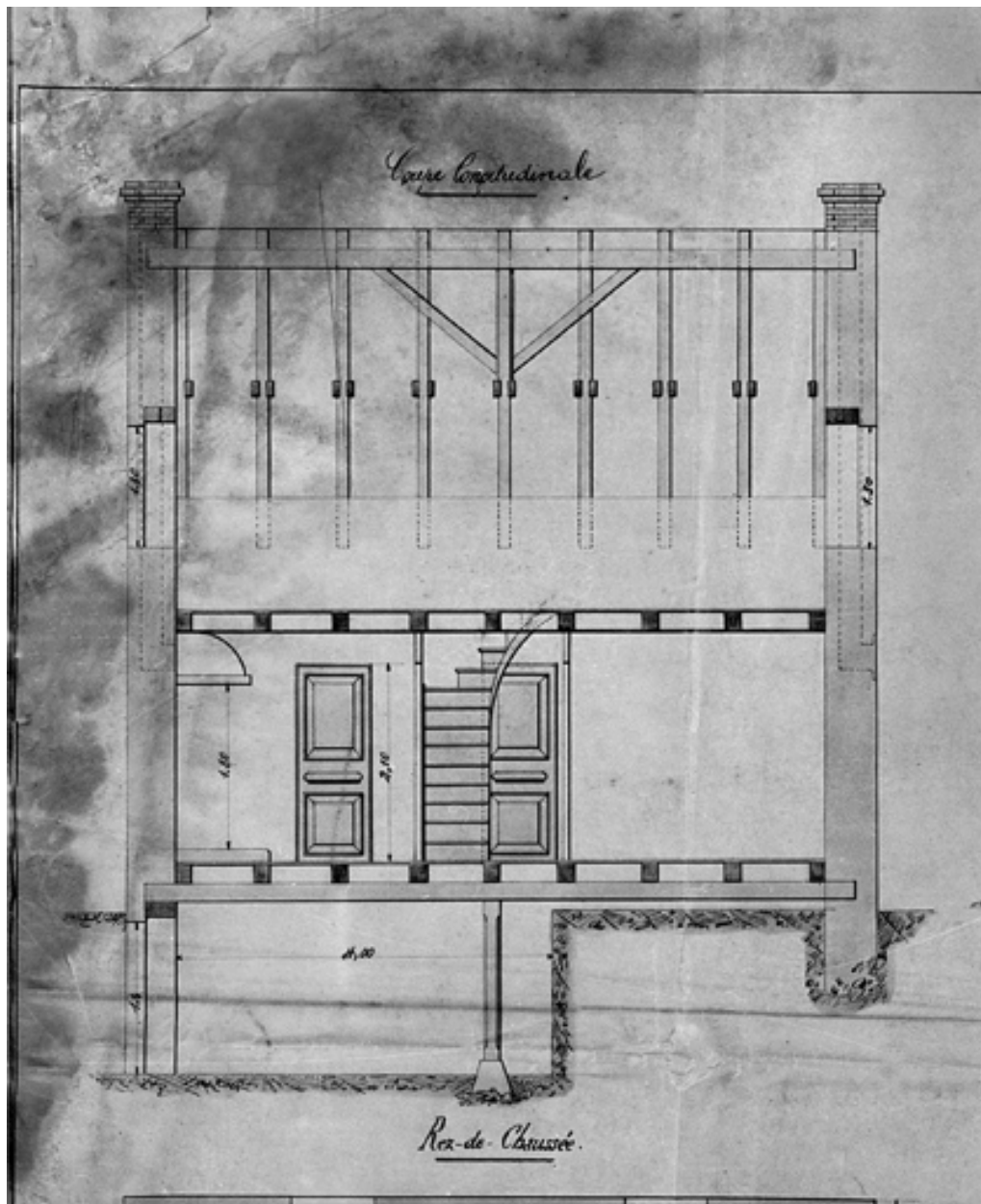
Habitation ouvrière. Cité Chatelot [coupe longitudinale].
