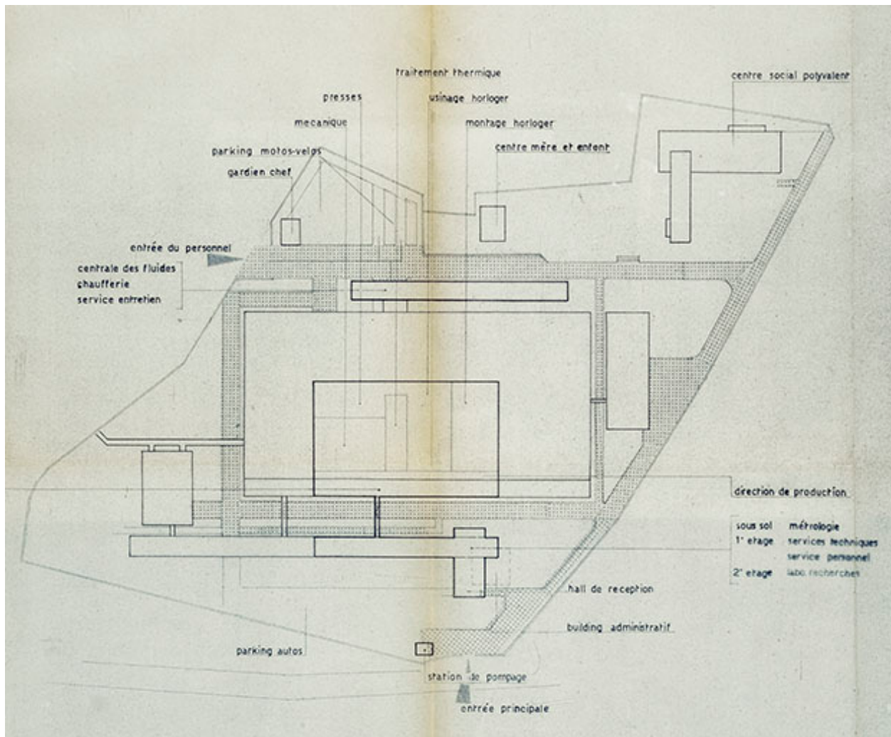
Plan-masse de l'usine, 1957.
