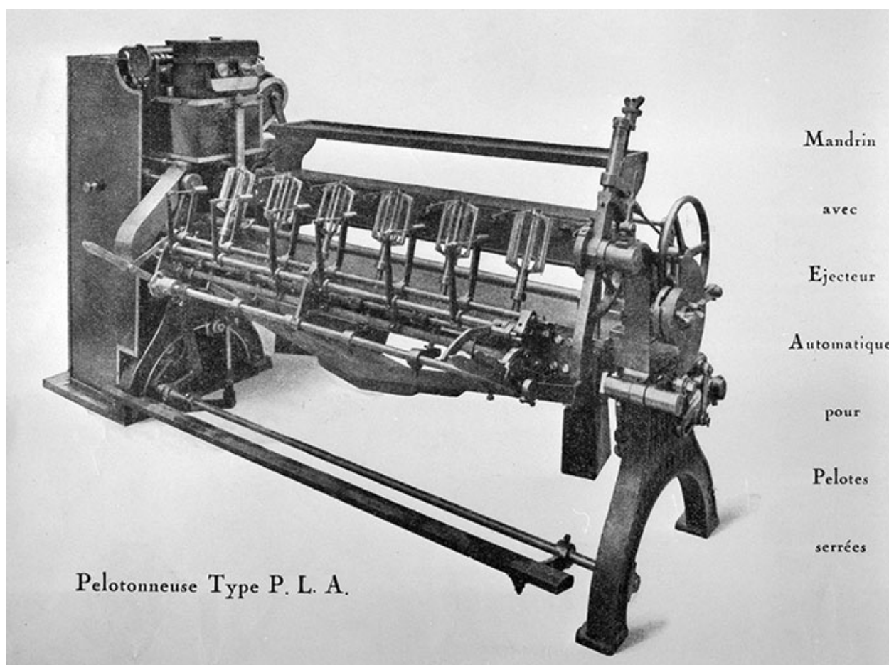
Pelotonneuse automatique type P.L.A.
