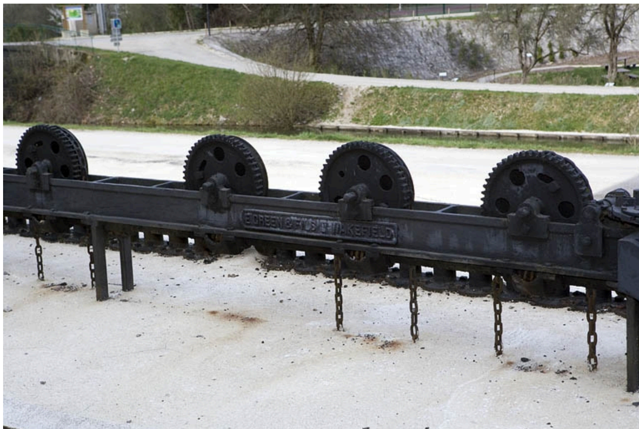
Détail des engrenages du système de levage des portes (?).
