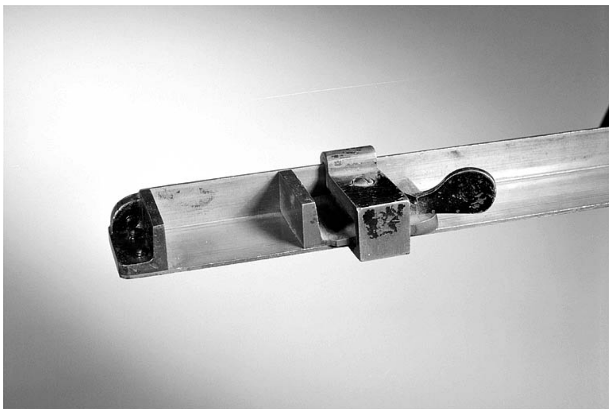
Blocage de l'équerre de l'un des composteurs métalliques : système à levier à axe vertical.
