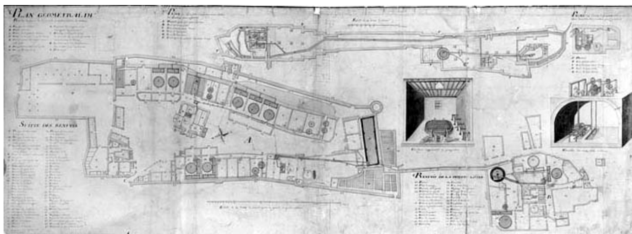
Plan géométral du Rets de chaussée de la grande et petite Saline de Salins.
