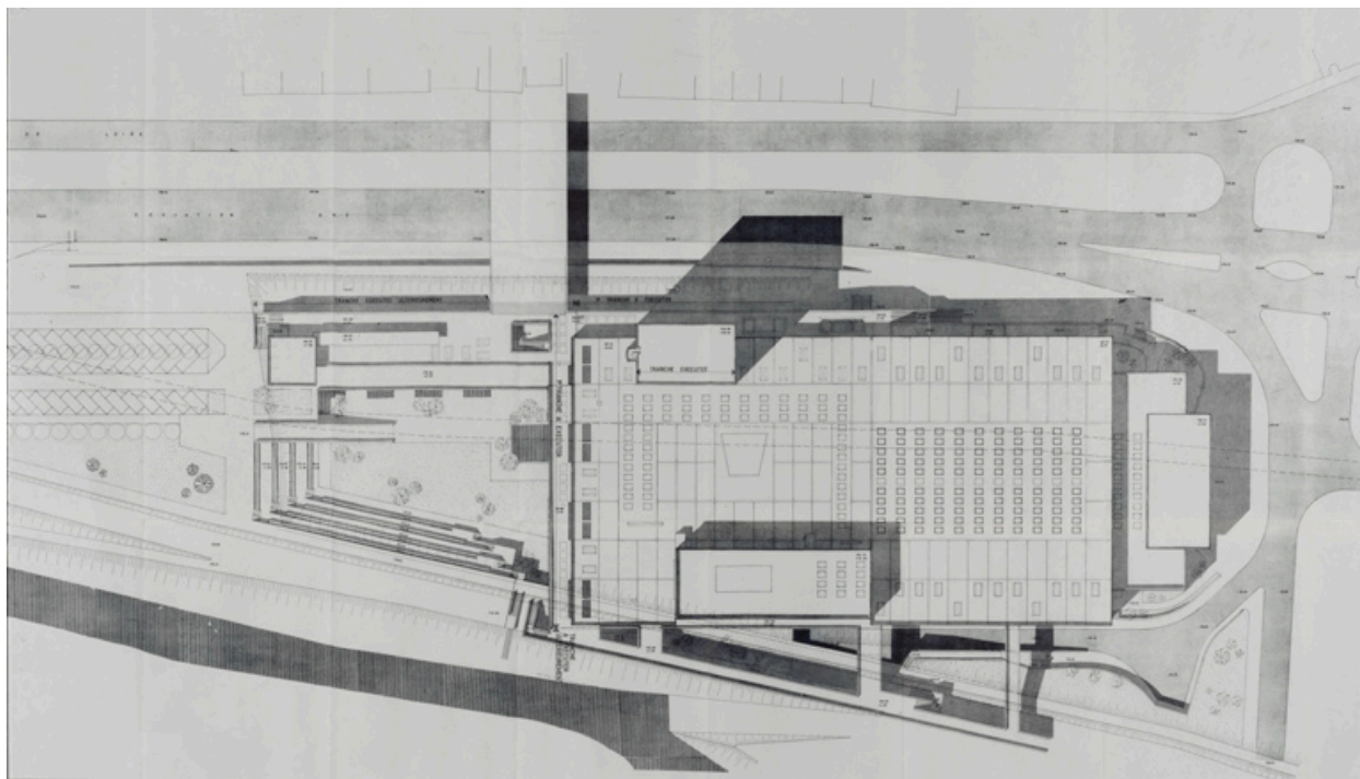
Nevers Centre municipal. Maison de la culture. 1. Plan d'ensemble [détail]. Octobre 1964, rect. novembre 1964.
