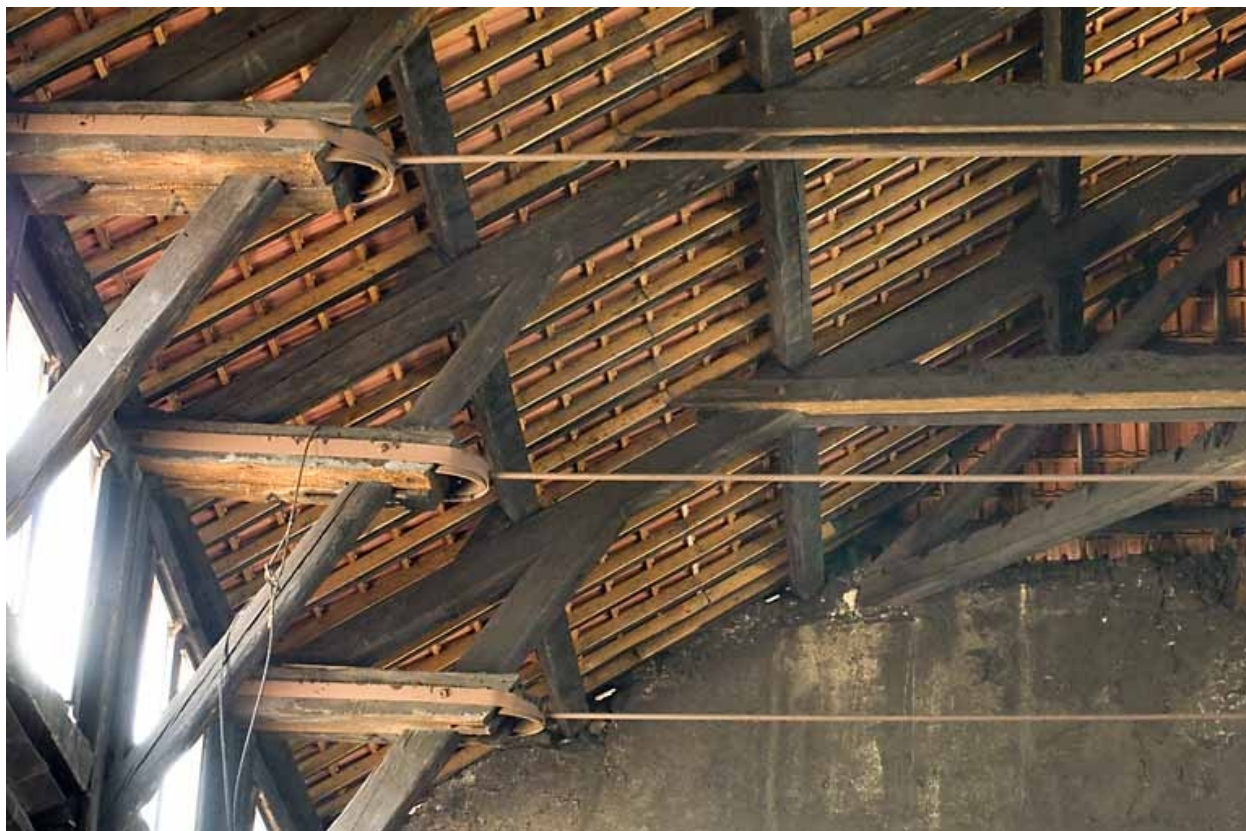
Atelier de fonderie. Détail des étriers de la charpente.
