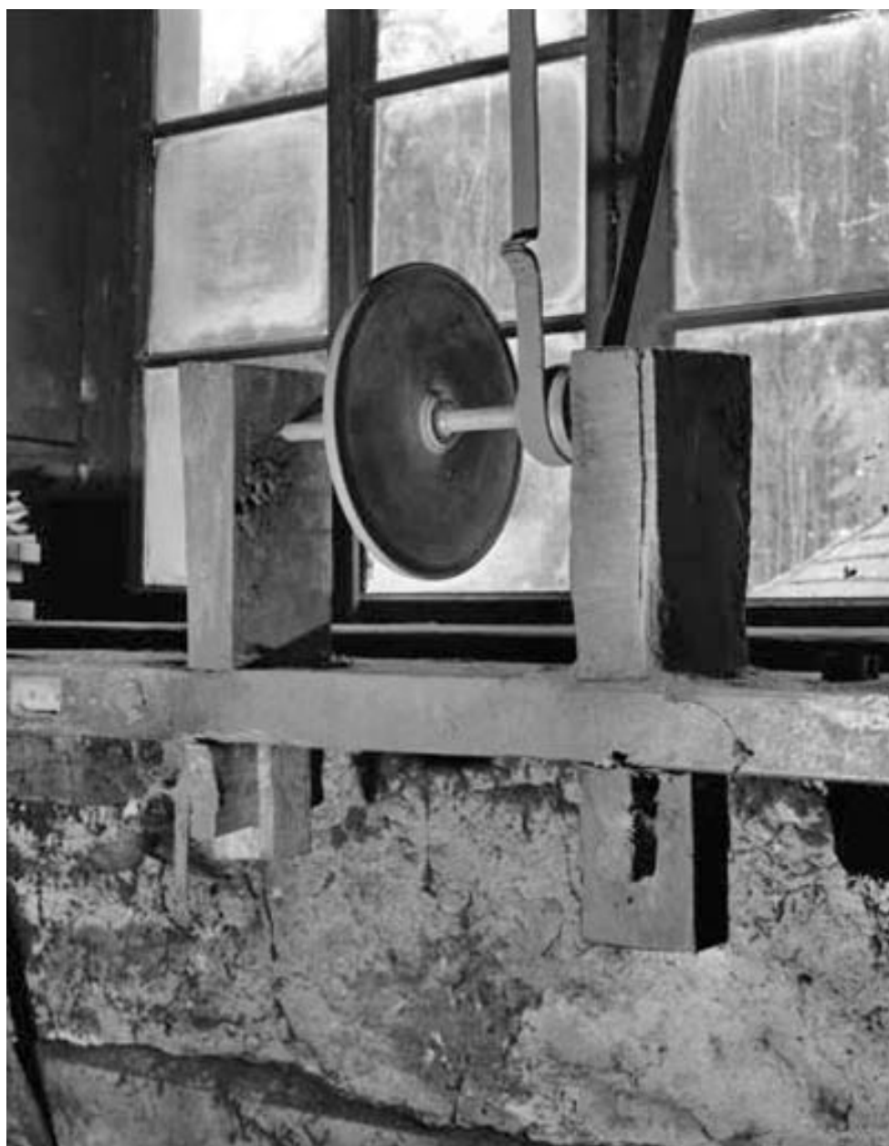
Intérieur : tour à polir.
