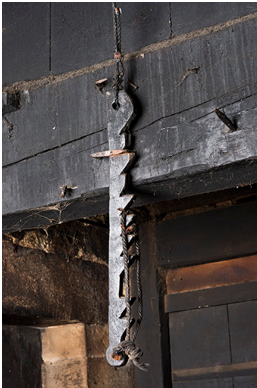
Grand tué : système de fermeture des volets.
