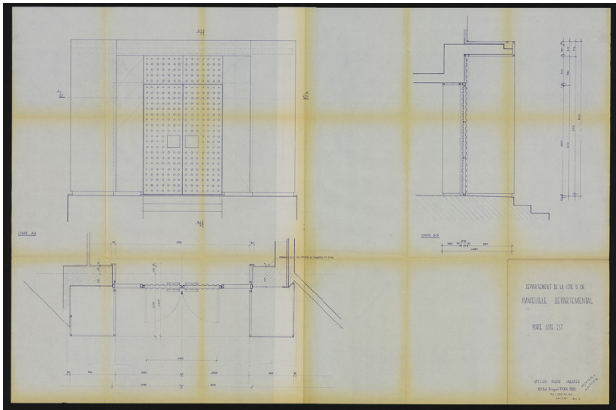
Façade antérieure nord : élévation, plan et coupe de la porte côté est, s.d., ca.1979. (Archives départementales de la Côte-d'Or, Dijon, 32 J 107)
