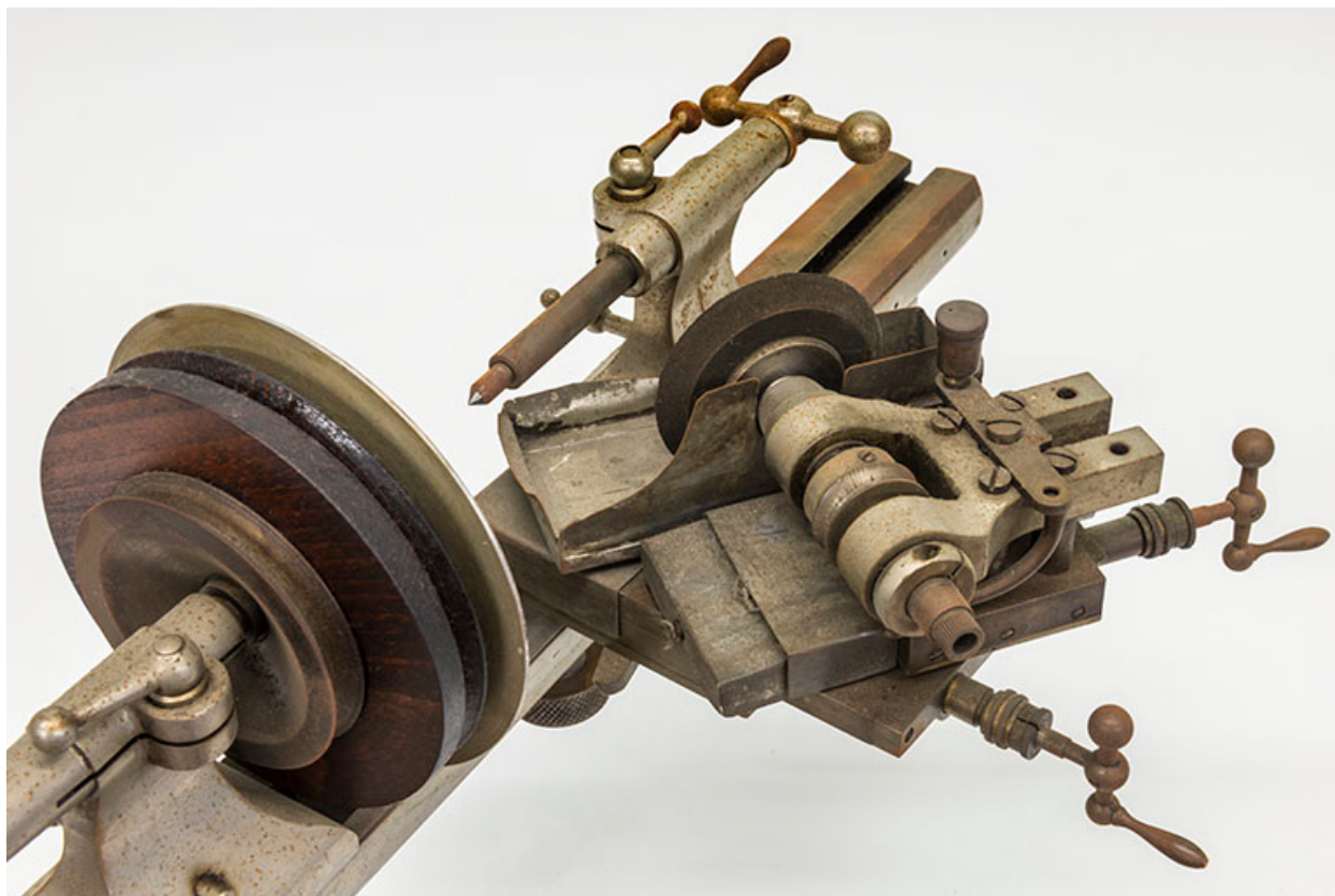
Détail du touret d'affûtage.
