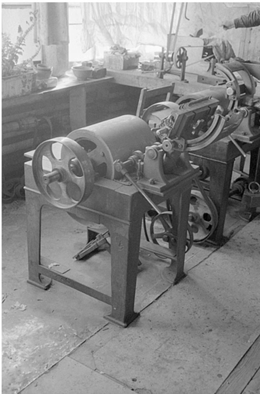
Appareil à cylindre. Porte-pierres levé.
