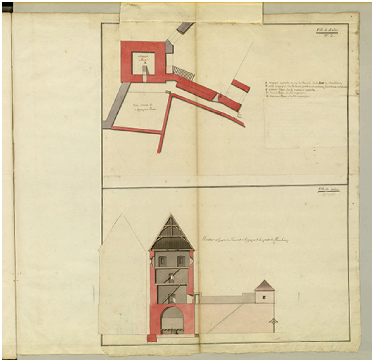
Folio 14. Ville de Salins. Tour et magasin à poudre de la porte de Chamboinoz. N°3. Plan, coupe et élévation. Magasin à poudre.
