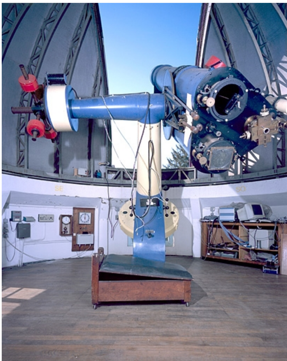
Vue d'ensemble de l'astrographe, devant la coupole ouverte.
