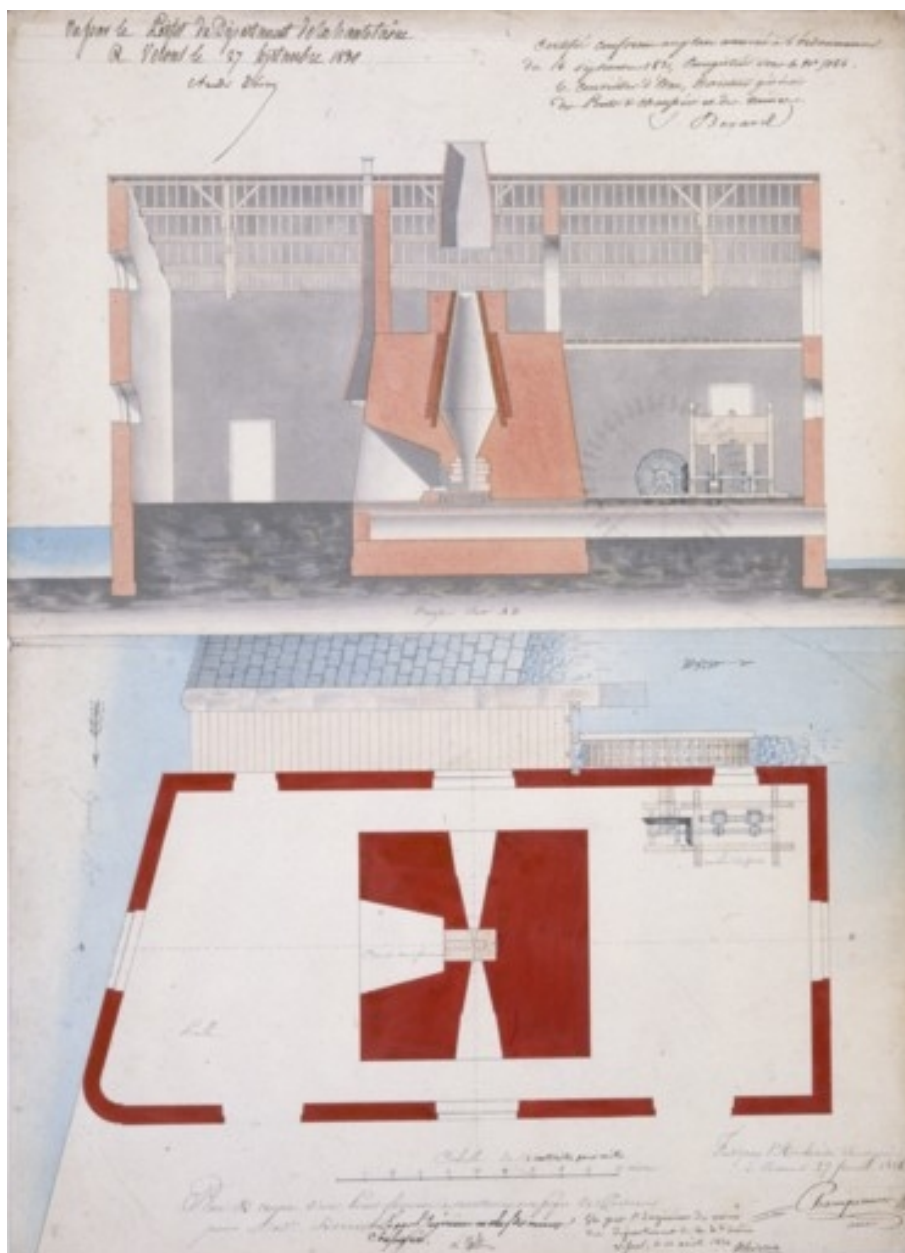
Plan et coupe d'un haut fourneau à construire aux forges de Pesmes.
