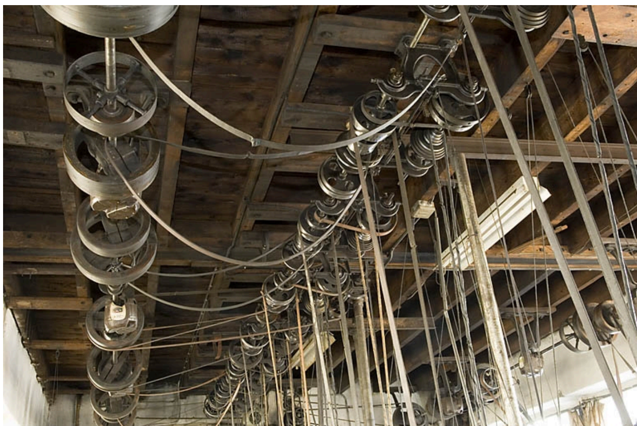
Poulies et courroies en cuir du système de transmission.
