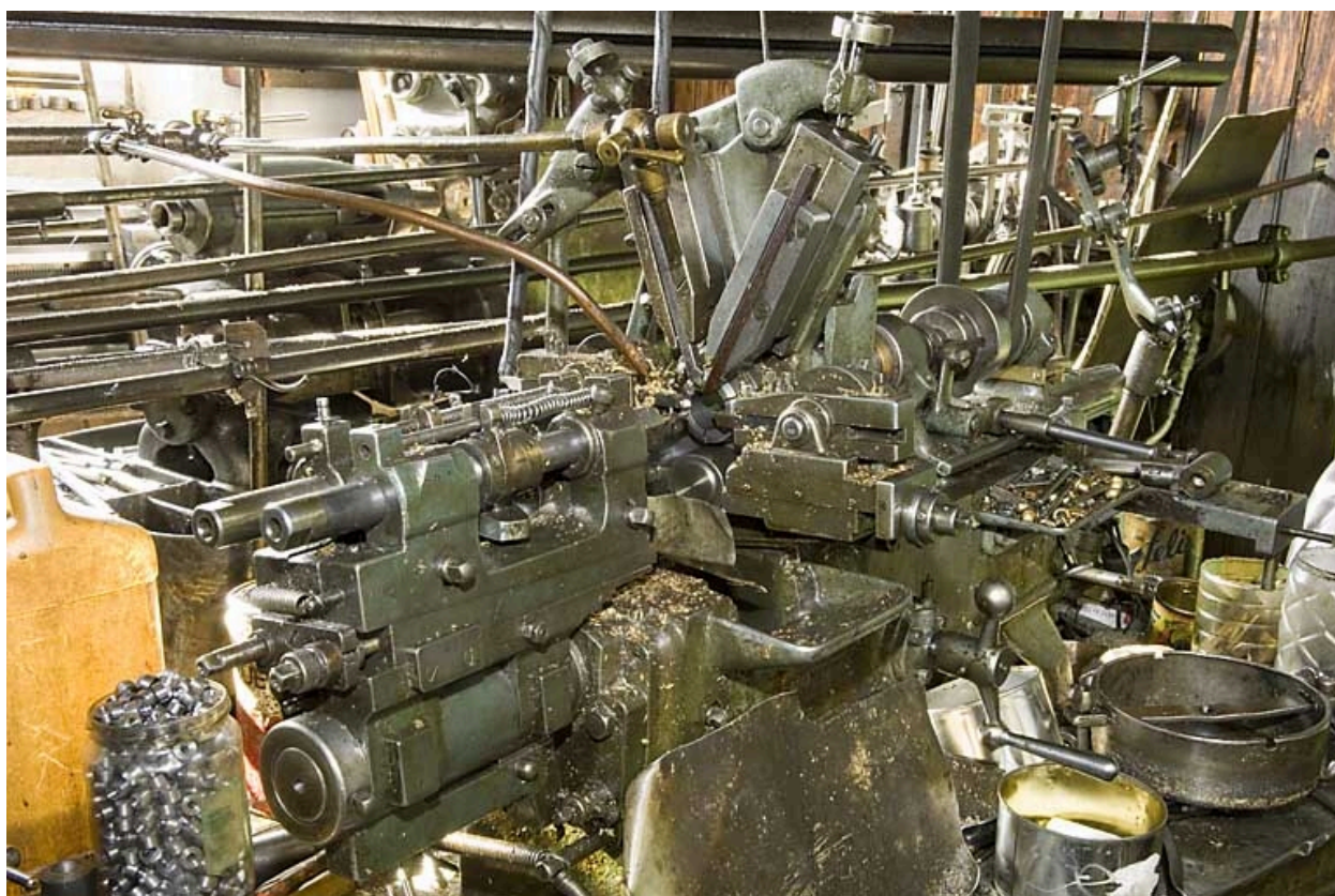
Détail d'un tour à décolleter Petermann (M).
