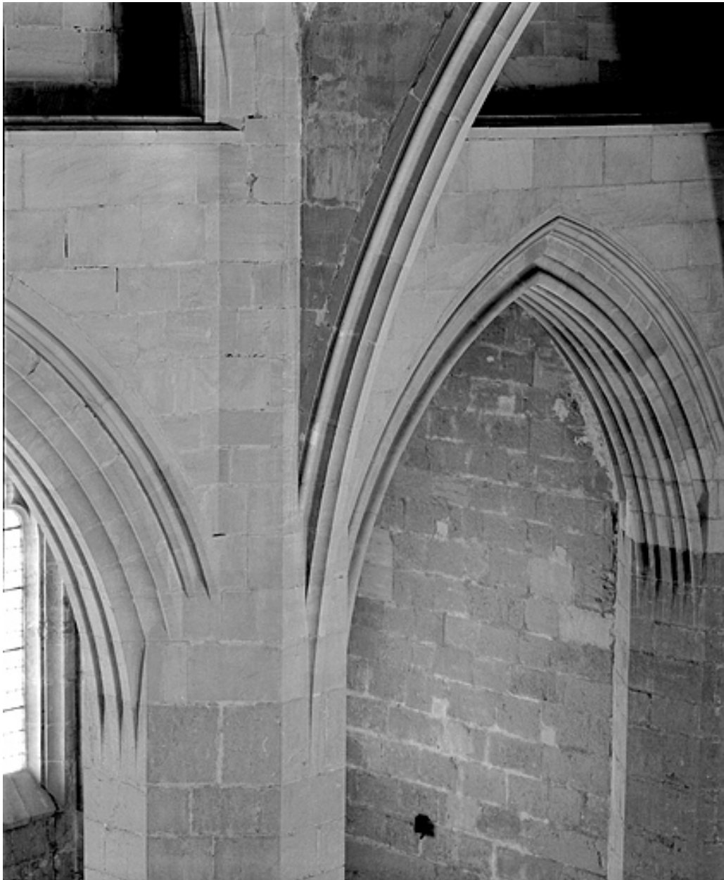
Retombée de l'ogive-diaphragme du vaisseau central sur la pile VIIN.
