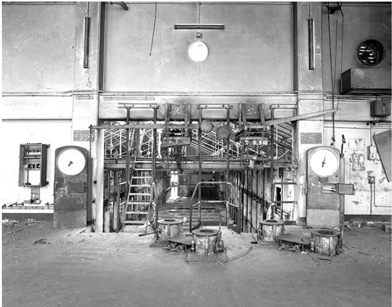
Balances du centre de commande des filatures tergal et nylon [TF1 et NF1 à 3].
