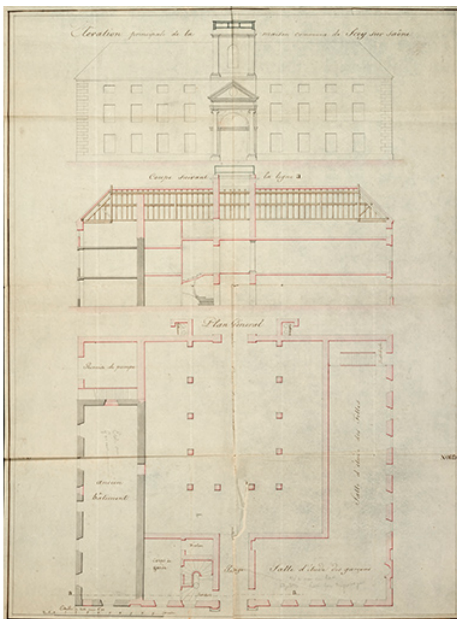
Élévation principale de la maison commune de Scey-sur-Saône. Coupe. Plan général [du rez-de-chaussée]. [1831].
