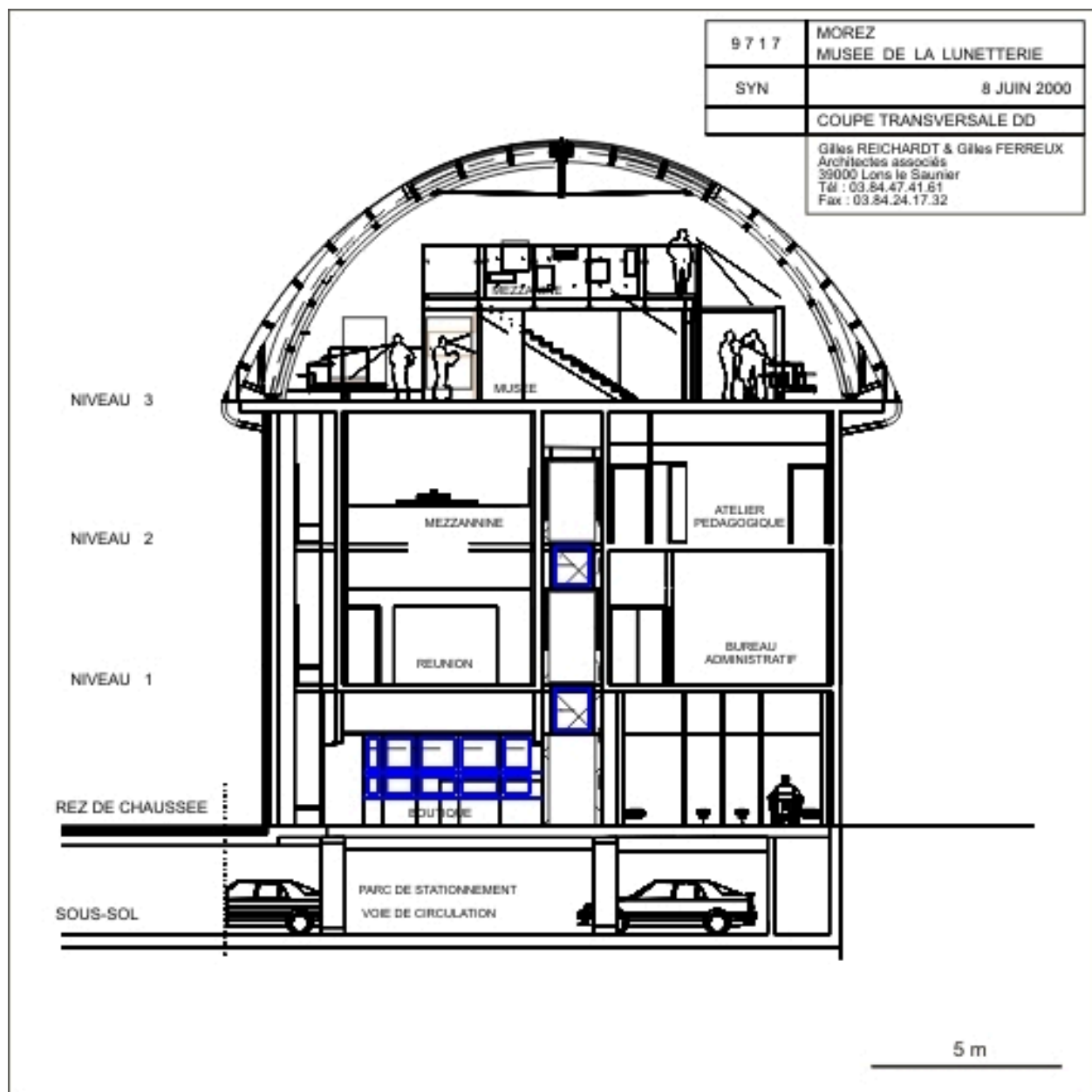
Coupe transversale DD, 2000.
